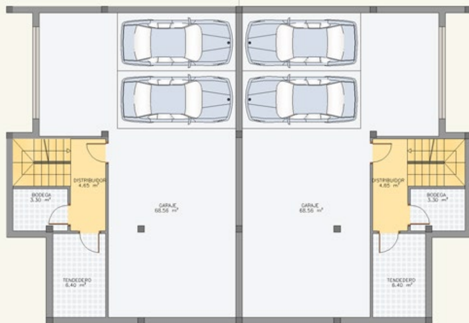
PLANTA SÓTANO
